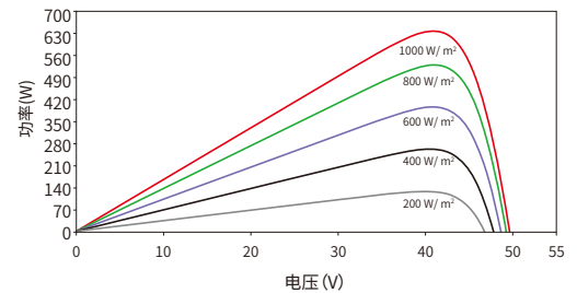
功率-电压曲线 66HL4M-BDV 635W
